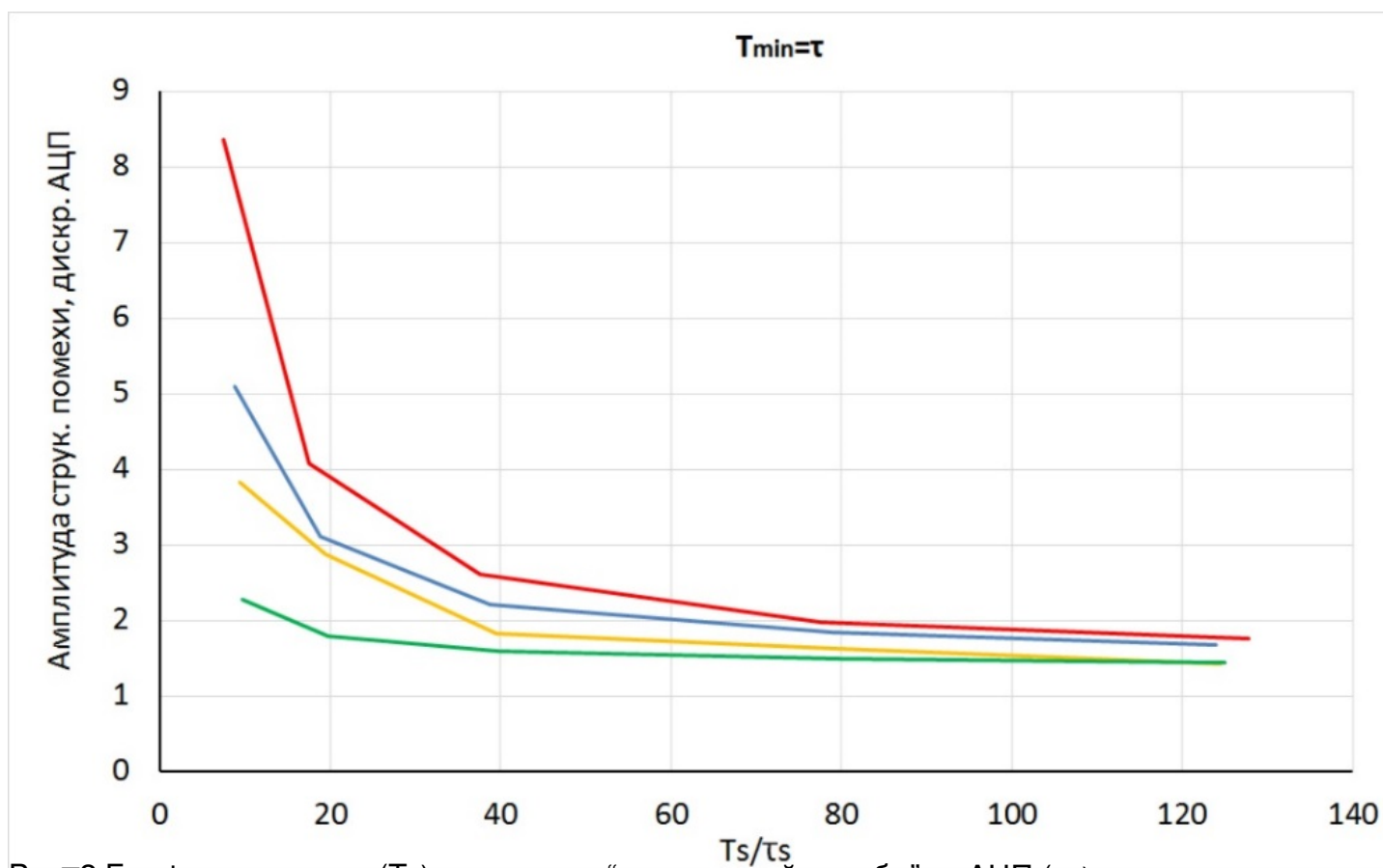
Рис. 29. Зависимость амплитуды дискретной структурной помехи от АЦП от отношения T_s/t_s при T_{min} = \tau
