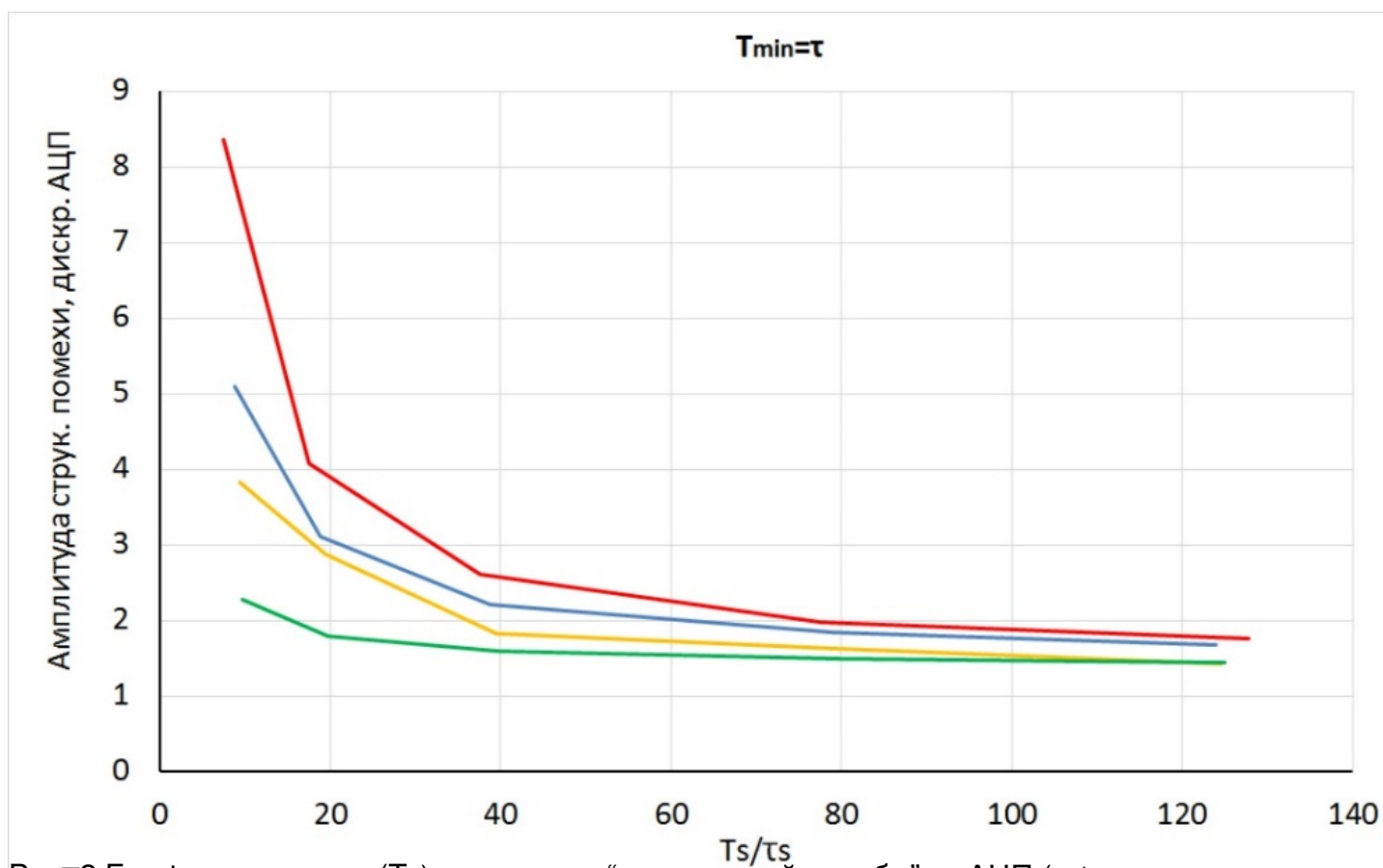
Рис. 2. Зависимость амплитуды дискретной помехи от отношения периода дискретизации к периоду сигнала. Расчет выполнен для T_{min} = \tau .
